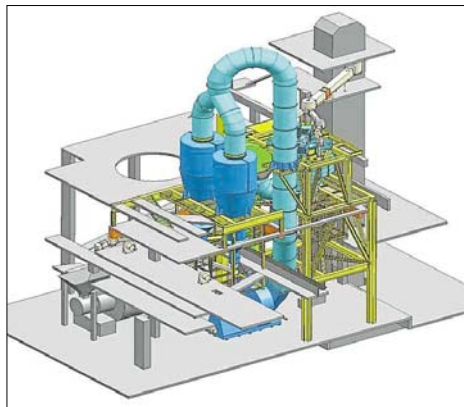
Die Darstellung zeigt, auf welchem Raum die neue Anlage in das bestehende Gebäude (grau) eingepasst wurde. Grafik: Pfeiffer
